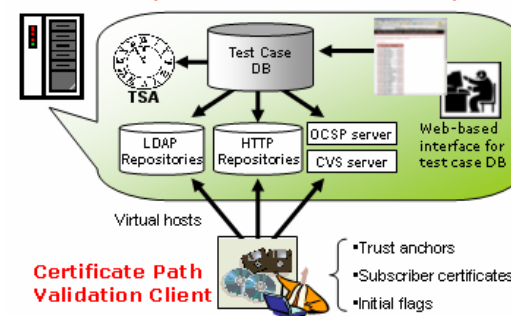
PKI Test Suite 2.0: Overview
